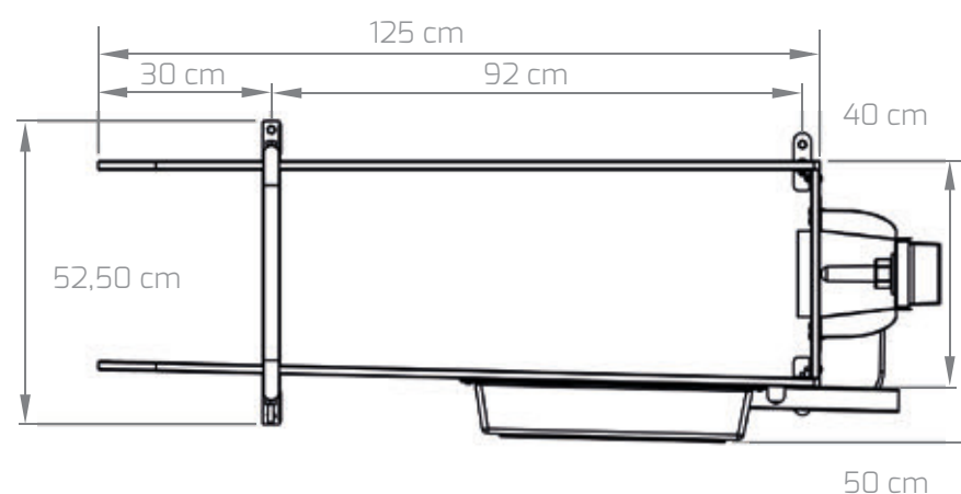
Bovenaanzicht
